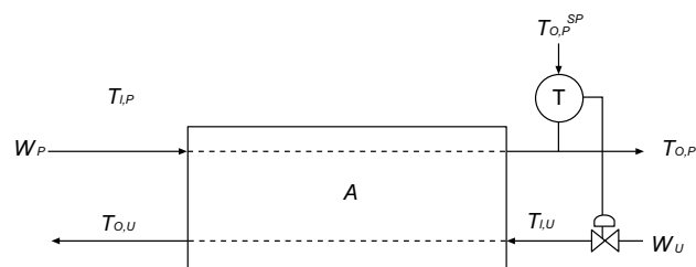
Fig. (3). Actual heat exchanger setup.
